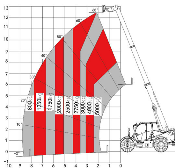
50THCJ13-CU1 载荷曲线图 Lifting diagram
