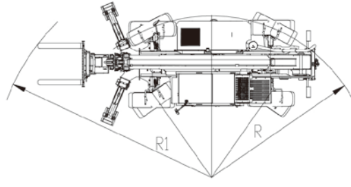
■ 前支腿支撑
