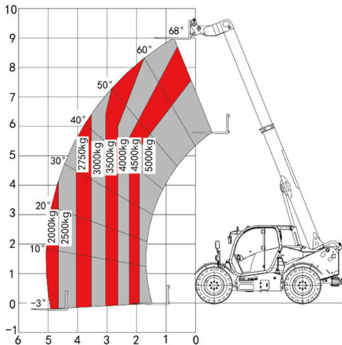
50THCJ09-CU1 载荷曲线图 Lifting diagram
