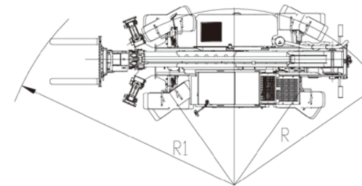
■ 前支腿抬起
